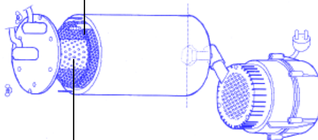
Tubo anódico baja polarización Anodic tube low polarisation Cod. RT011390 Tubo anódico standard Anodic standard tube Cod. 1R011382
