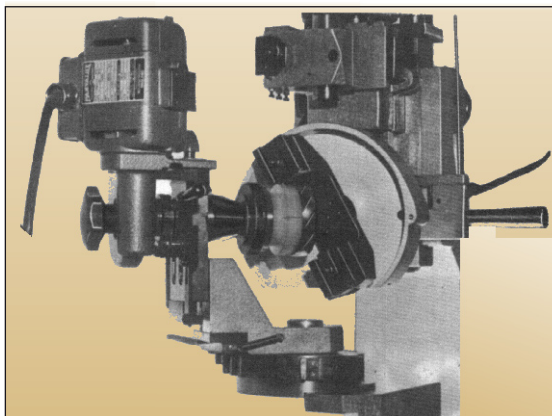
M-2 con soportes divisor y lupa (cod. SF032000) para cortes circunferenciales en brazaletes con divisor y motorización (cod. SF032110). M-2 with divider and scope supports (cod. SF032000) for florentine work in bangles with divider and motorized drive (cod. SF032110).
