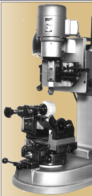
M-2 con accesorios brazaletes y cabezal vertical (cod. SF030400). M-2 with accessories for bangles and vertical head (cod. SF030400).
